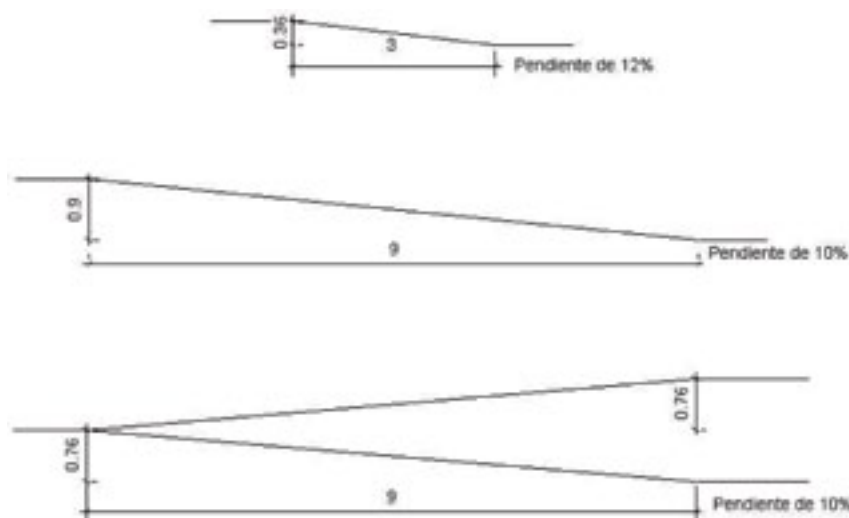
Figura 8 - Pendiente longitudinal en función de la extensión.
