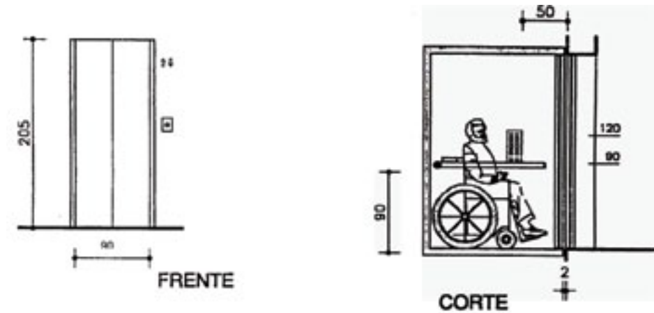
Figura 19 – Medidas de la cabina del ascensor.
