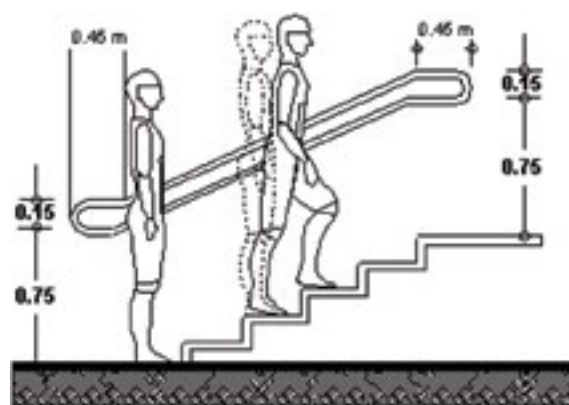
Figura 13. Dimensiones de los pasamanos para escaleras.
